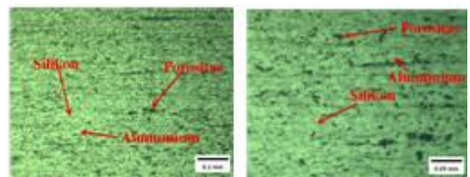
Gambar 13. Struktur Mikro pada spesimen temperatur 250°C tepi kiri
