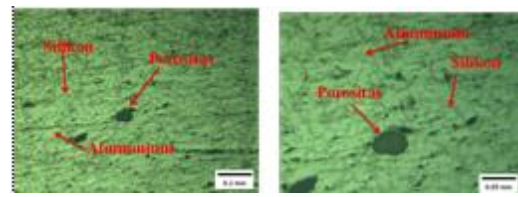
Gambar 14. Struktur Mikro pada spesimen temperatur 300°C tepi kanan
