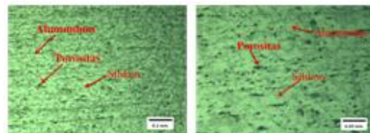
Gambar 8. Struktur Mikro pada spesimen temperatur 200°C tepi kanan
