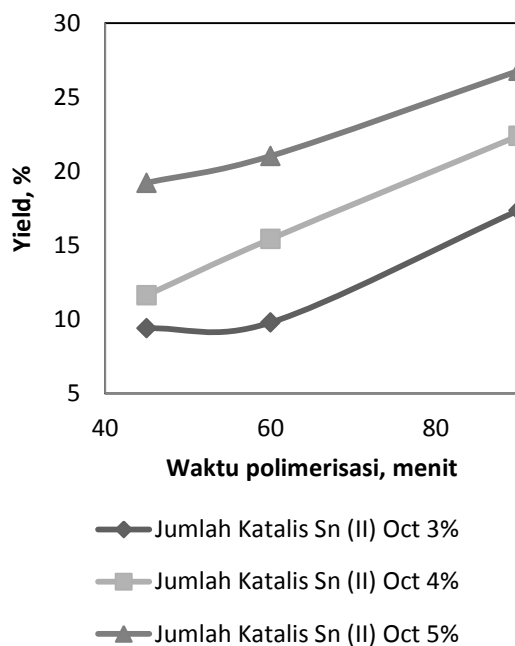
Gambar 2. Hubungan antara waktu polimerisasi dan yield PLA pada berbagai jumlah katalis
