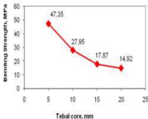
Gambar 3. Kurva kekuatan bending komposit sandwich.
