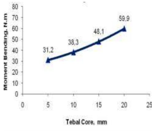
Gambar 2. Kurva momen bending komposit sandwich.
