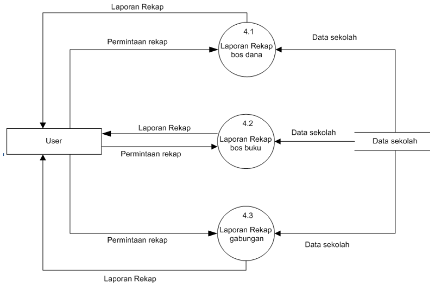
Gambar 7. Diagram Alir Data Level 2 Proses Pelaporan Rekap Penerima BOS
