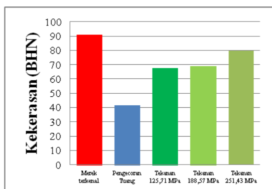
Gambar 11. Grafik kekerasan
