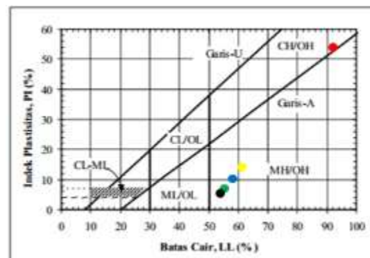
Gambar 3. Sistem Klasifikasi Tanah Sistem Unified
