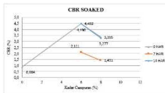
Gambar 6. Perbandingan Nilai CBR Terendam Pada Variasi Tanah Asli + 6% Serbuk Gypsum dan Tanah Asli + 8% Serbuk gypsum Dengan Curing Dan Tanpa Curing
