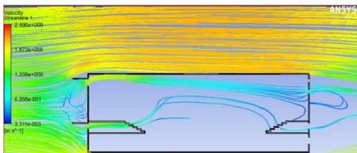
Gambar 7. Analisa overhang langsung di atas bukaan
