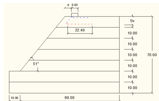
Gambar 6 Contoh model lereng dengan perkuatan geotekstil
