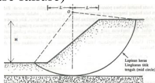
Gambar 3 Tipe keruntuhan di bawah kaki lereng (Sumber : Das, B.M. 2009:177)
