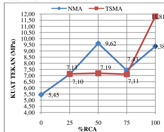
Gambar 4. Grafik Rekapitulasi Kuat Tekan Rata-rata Silinder Beton Porous
