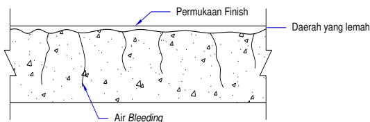
Gambar 9. Bleeding yang terjadi balok balok beton.
