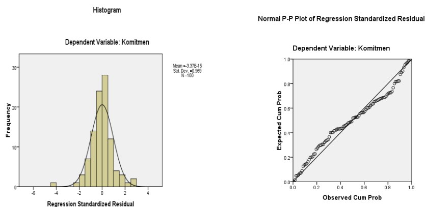
Gambar 8. Histogram peluang normal
