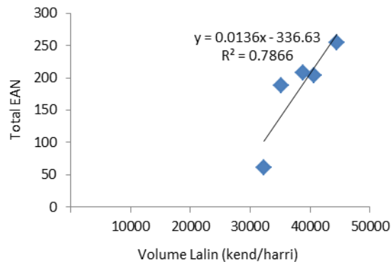
Gambar 4. Grafik Hubungan Volume Lalin Dengan Total EAN
