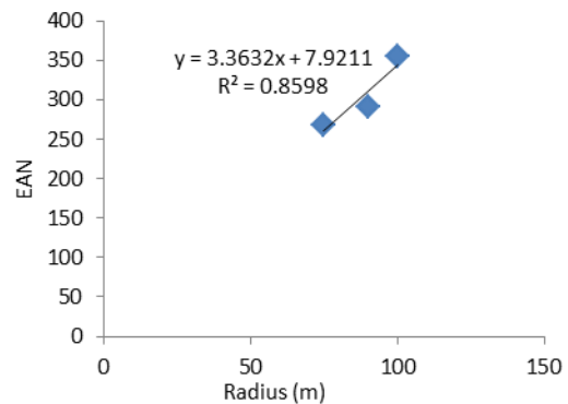
Gambar 3. Grafik Hubungan Radius Dengan EAN
