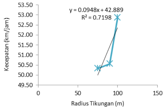
Gambar 5. Grafik Hubungan Radius Dengan Kecepatan Kendaraan
