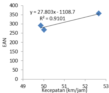
Gambar 2. Grafik Hubungan Kecepatan Dengan EAN
