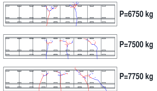
Gambar 9. Pola retak benda uji a_2b_2c_2d_1
