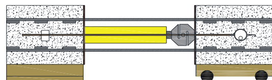
Gambar 3. Skema Pengujian Pull Out
