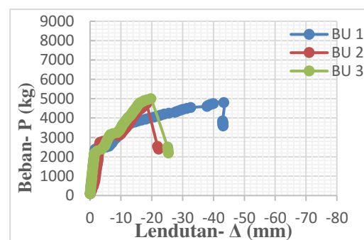
Gambar 6. Grafik hubungan P- \Delta benda uji a_2b_1c_1d_1
