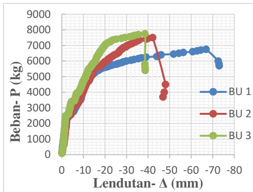
Gambar 7. Grafik hubungan P- Δ benda uji a_2b_2c_2d_1
