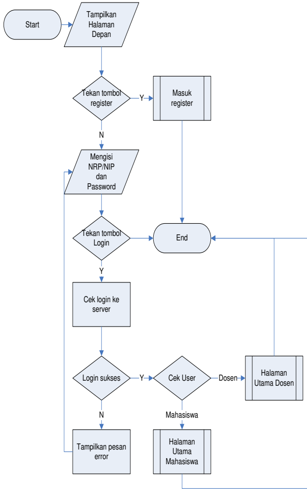
Gambar 1. Gambaran Aplikasi Secara Umum
