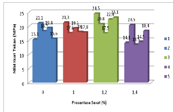
Gambar 2. Diagram Batang Hasil Kuat Tekan Beton Ringan tanpa Pelapis
