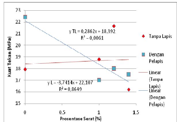
Gambar 6. Grafik gabungan kuat tekan rata-rata beton ringan tanpa lapis dengan beton ringan berlapis
