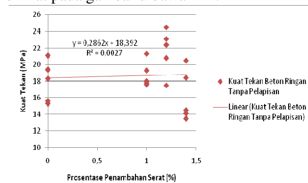
Gambar 4. Grafik Regresi Hubungan Prosentase Serat Bambu dengan Kuat Tekan Beton Ringan Tanpa Pelapisan Batu Apung
