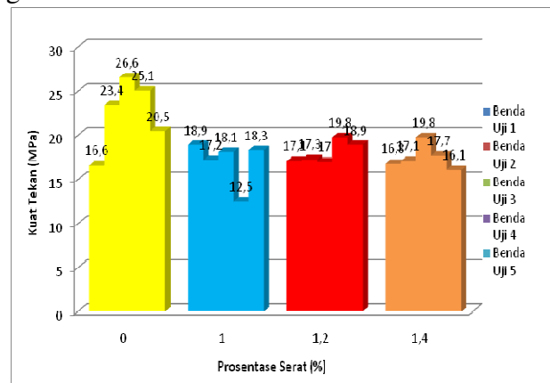
Gambar 3. Diagram Batang Kuat Tekan Beton Ringan dengan Pelapis
