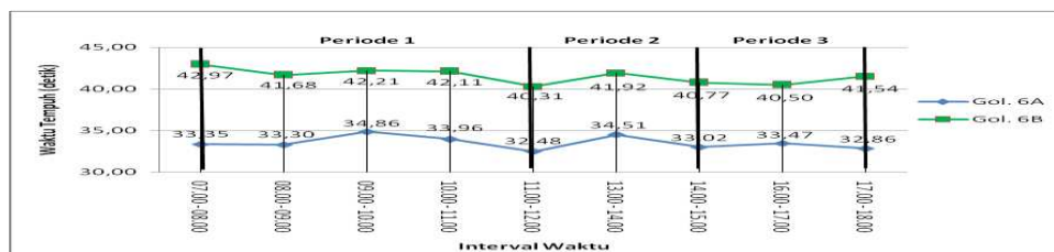
Gambar Waktu Tempuh Rata-Rata Kendaraan Gol. 6A dan 6B pada Ruas Jalan Semarang-Kendal Km 22 sampai Km 25.
