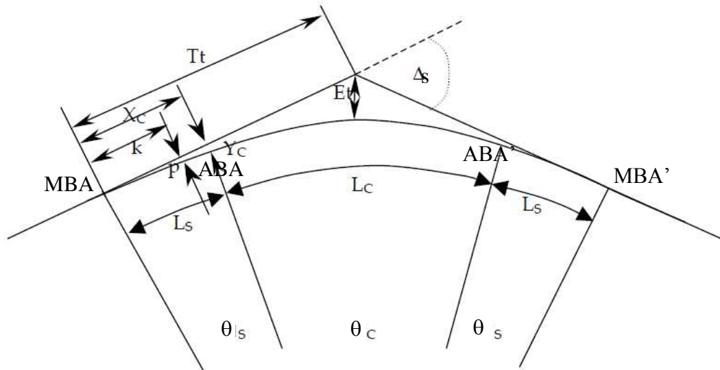
Gambar 1. Lengkung Horizontal
