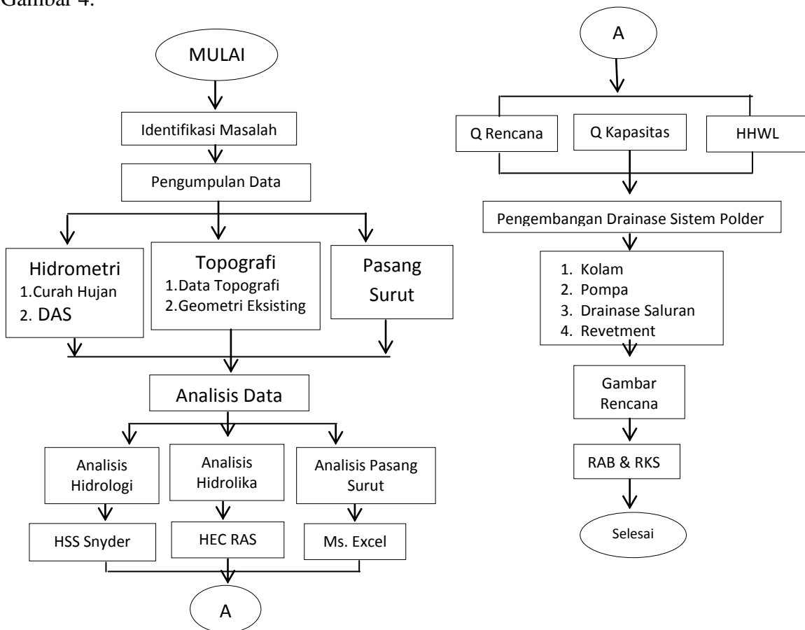
Gambar 4. Bagan Alir Metode Pengembangan Drainase Sistem Polder Sungai Sringin
