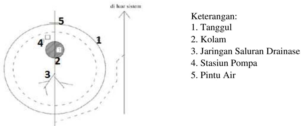
Gambar 2. Komponen Sistem Polder (Al Falah , 2008)
