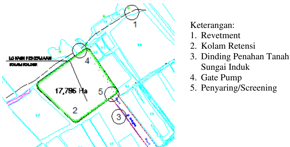
Gambar 8. Layout Rencana Sistem Drainase Sistem Polder Sungai Sringin
