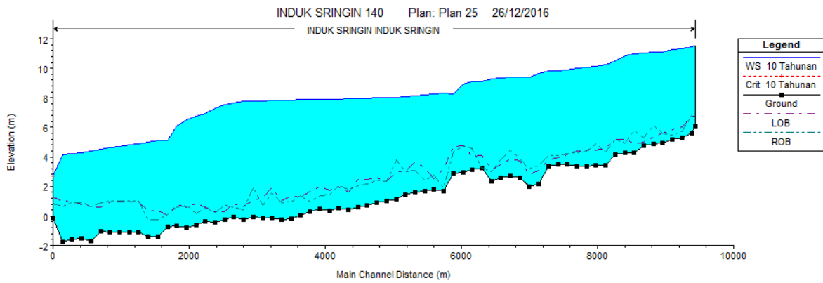
Gambar 5. Tampilan Hasil Analisis Steady Flow Profil Memanjang Saluran Kondisi Eksisting
