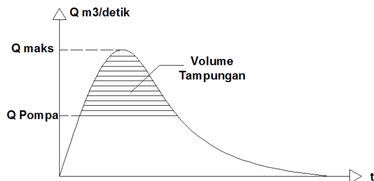
Gambar 3 Volume Tampungan Kolam Berdasarkan Kapasitas Pompa dan Debit
