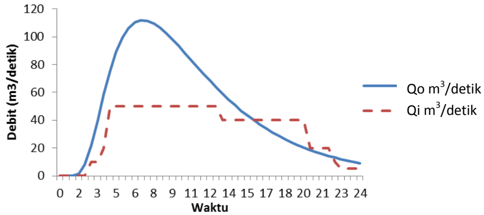
Gambar 7. Grafik Hubungan Q Inflow dan Q Outflow
