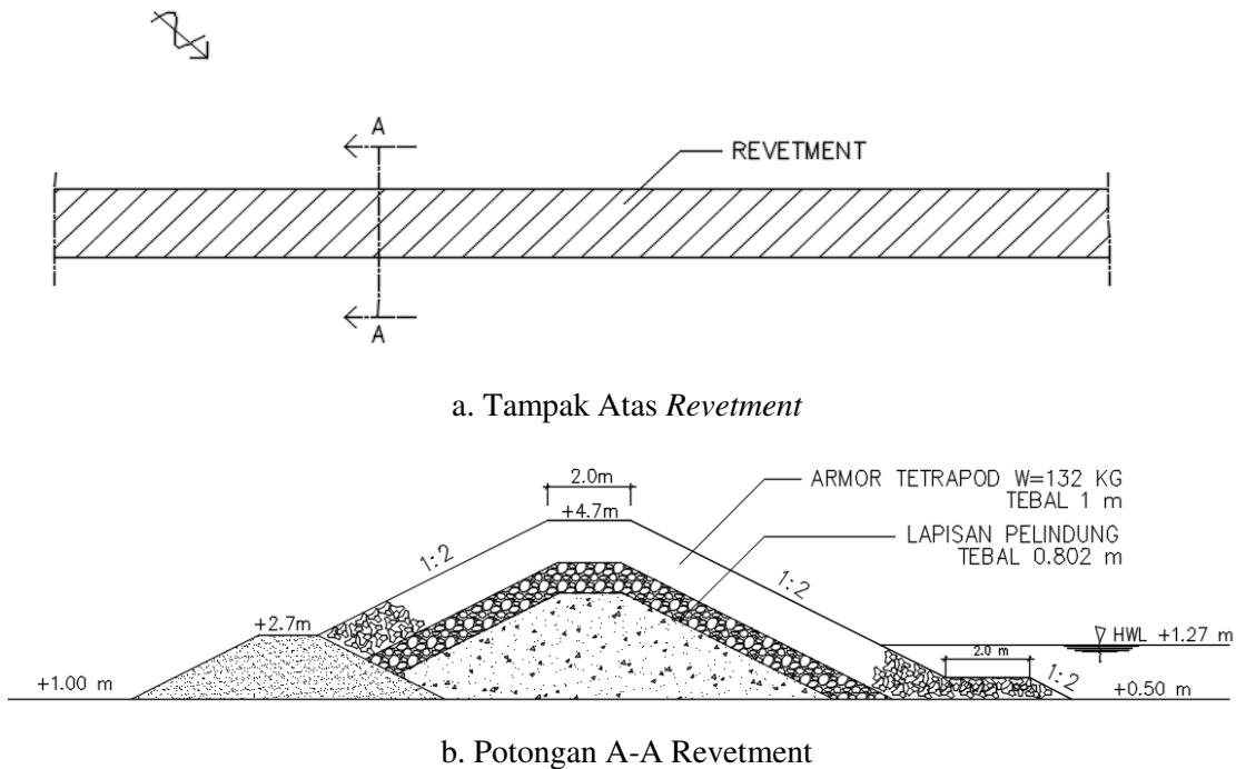
Gambar 11. Revetment
