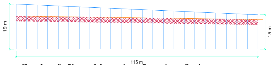
Gambar 9. Sketsa Memanjang Sepanjang Oprit
