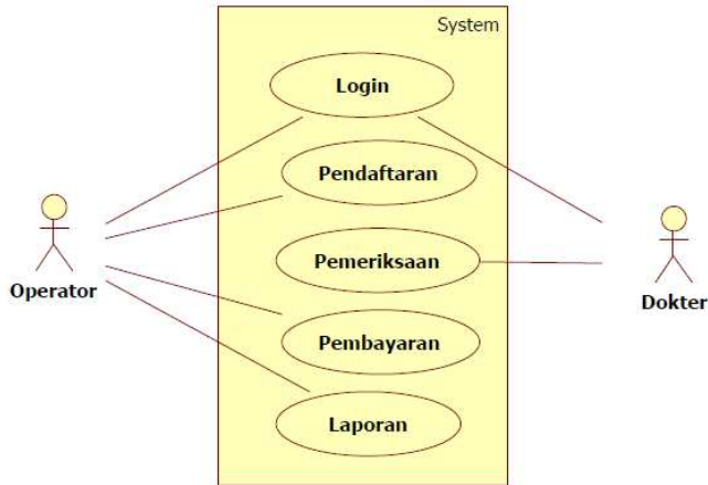
Gambar 2. Use Case Hak Akses Operator dan Dokter
