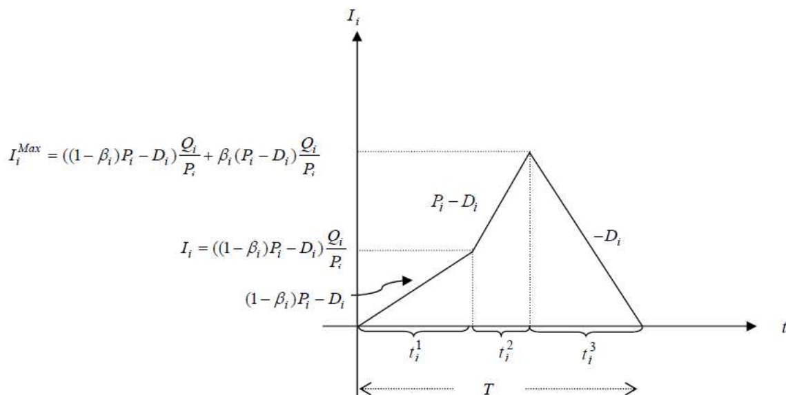
Gambar 1. EPQ multi produk mesin tunggal dengan pengolahan ulang dalam satu siklus
