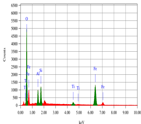
Gambar 4. Hasil analisis dengan EDX
