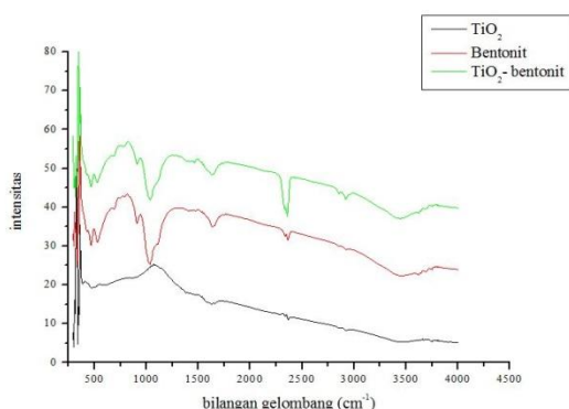
Gambar 1. Spektrogram TiO 2 , bentonit dan TiO 2 -Bentonit
