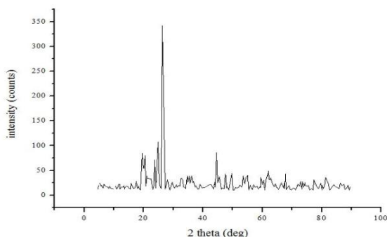
Gambar 2. Pola difraksi TiO 2 -Bentonit menggunakan XRD
