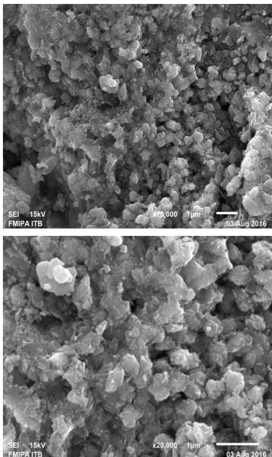
Gambar 3. Morfologi SEM \text{TiO}_2 bentonit perbesaran 10.000 kali (atas) dan 20.000 kali (bawah)
