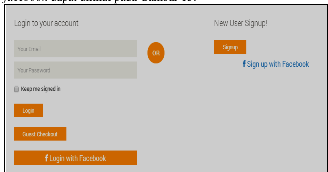
Gambar 14. Halaman Login
