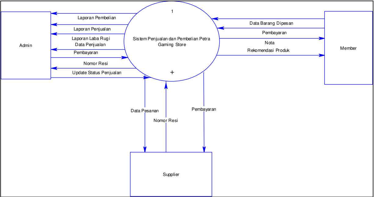
Gambar 1. Konteks Diagram
