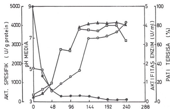
Gambar 1. pH medium (o), aktifitas glukamilase ( \blacktriangle ), aktifitas spesifik glukamilase ( \square ) dan pati tersisa ( \bullet ) dalam medium setelah fermentasi oleh R. oryzae .
