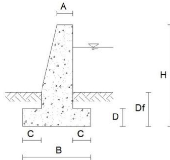
Gambar 5. Dimensi Penampang Parapet Beton
