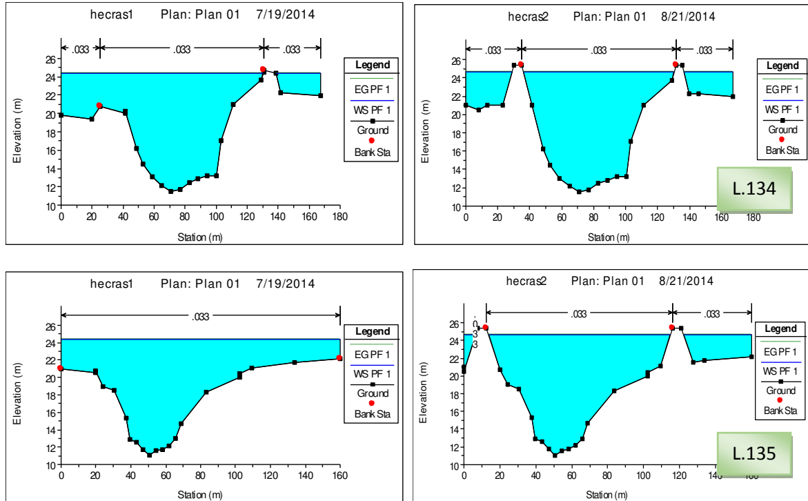
Gambar 3. Kondisi Eksisting dan Perbaikan Penampang Sta 120, Sta 127, Sta 134 dan Sta135. (lanjutan)
