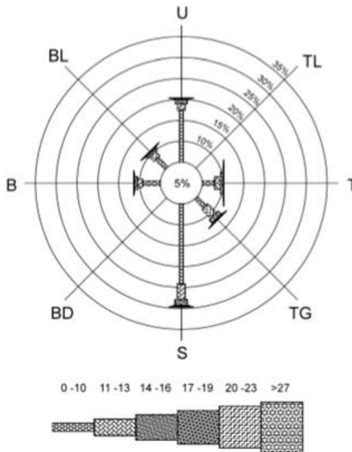
Gambar 2. Windrose Pantai Raja dari Tahun 1991-2014
