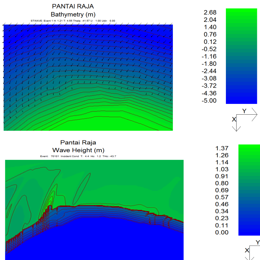
Gambar 7. Pemodelan penjalaran gelombang dengan program STWAVE (NEMOS)
