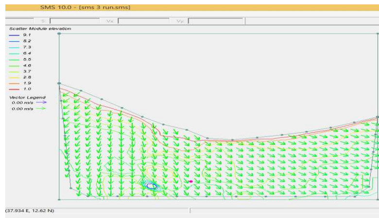
Gambar 5. Hasil running ADCIRC berupa pola vector
