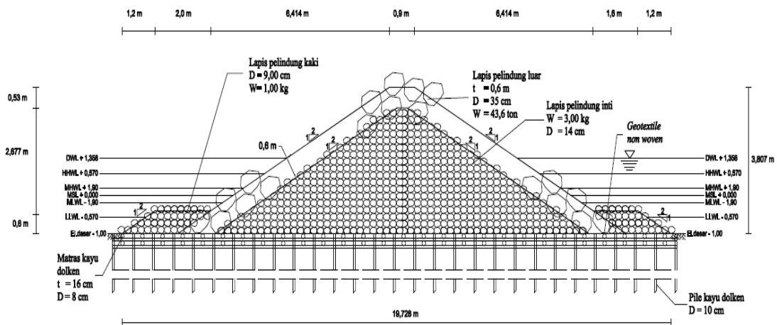
Gambar 11. Gambar desain potongan melintang groin rencana
