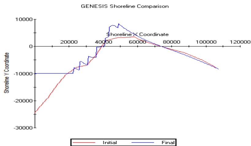
Gambar 8. Perubahan garis pantai dari tahun 2015 – 2020 hasil pemodelan GENESIS
