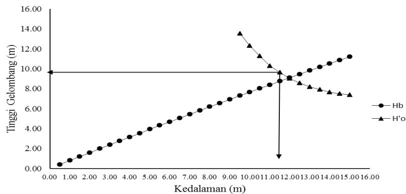
Gambar 4. Grafik penentuan lokasi gelombang pecah dengan gelombang maksimal kala ulang
