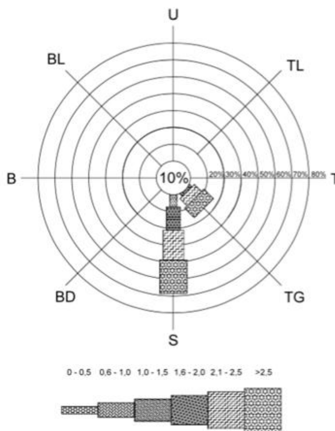
Gambar 3. Waverose Pantai Raja dari Tahun 1991-2014
