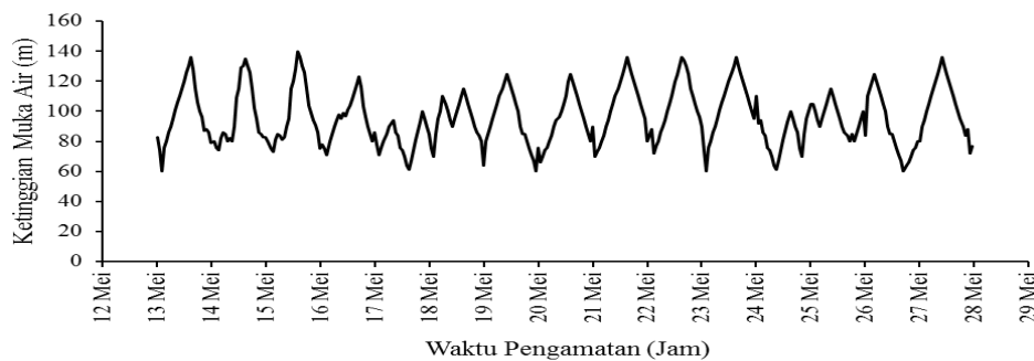
Gambar 1. Grafik pasang surut Pantai Raja Desa Sei Raja (Sumber : BMG Stasiun Meteorologi Maritim Iskandar Pangkalan Bun Tahun 2015)
