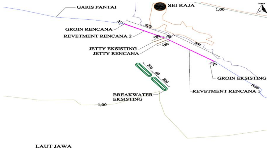
Gambar 9. Lokasi penempatan bangunan pelindung Pantai Sei Raja
