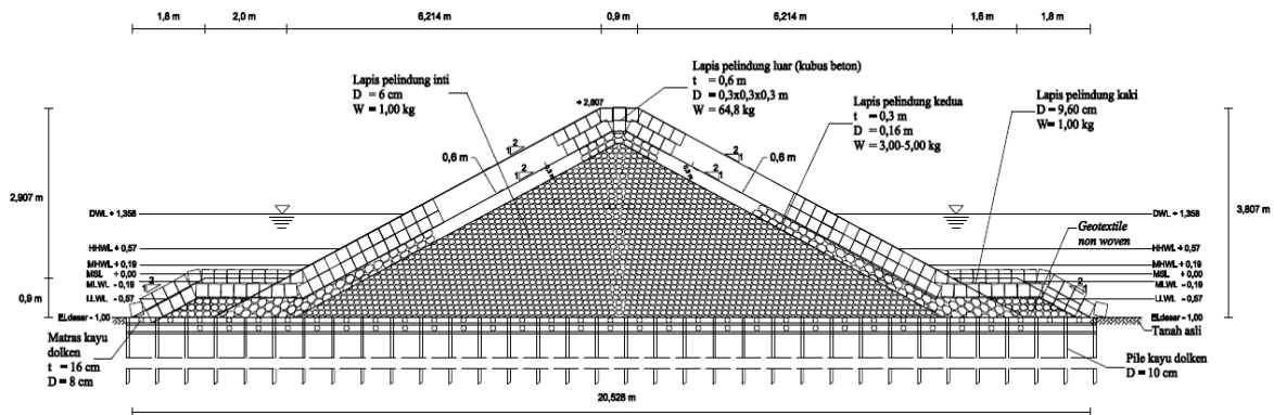
Gambar 12. Gambar desain potongan melintang jetty rencana
