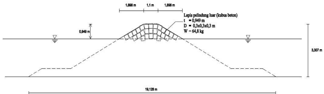
Gambar 10. Gambar desain potongan melintang rehabilitasi breakwater
