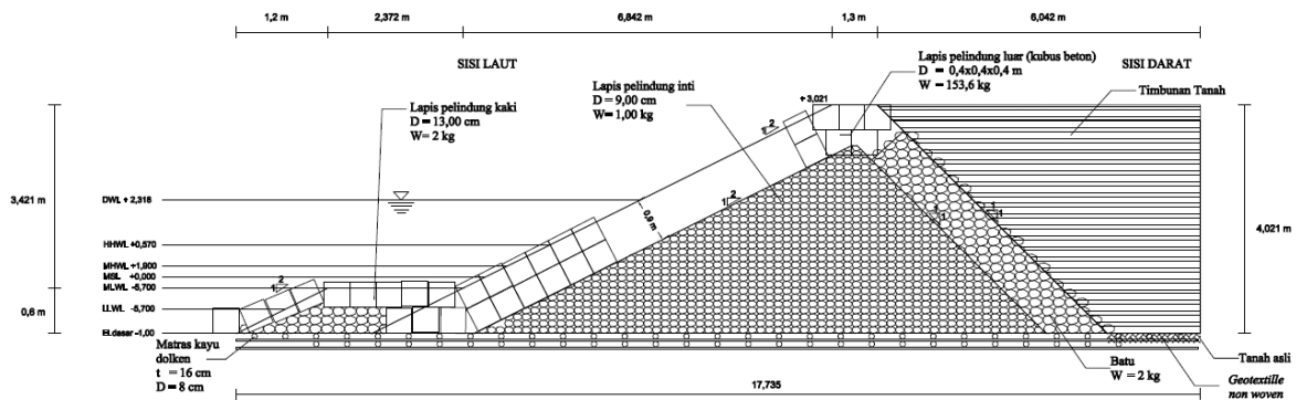
Gambar 13. Gambar desain potongan melintang revetment rencana sisi Barat dan Timur
