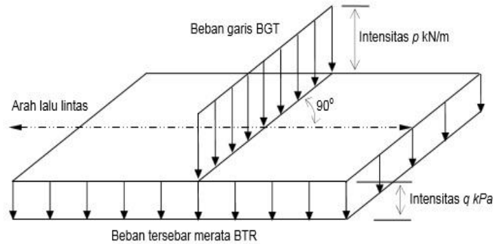
Gambar 2. Distribusi beban D dan beban KEL
