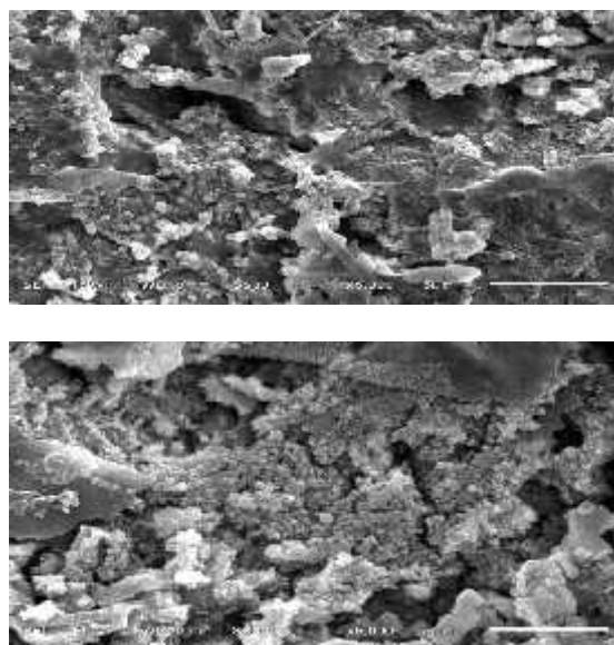
Gambar 7. Foto SEM spesimen baja lunak: (atas) tanpa dan (bawah) dengan KMK yang direndam dalam 0.25 M H_2SO_4 selama 3 hari pada suhu kamar
