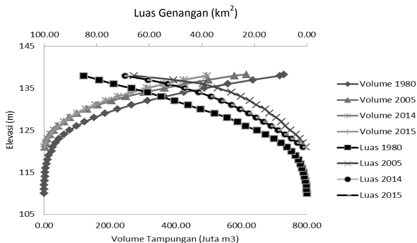
Gambar 2. Kurva Hubungan Volume Tampung- Luas Genangan – Elevasi
