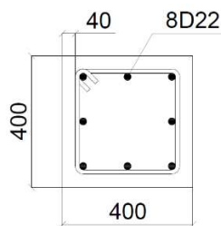
Gambar 12. Penampang tiang pancang
