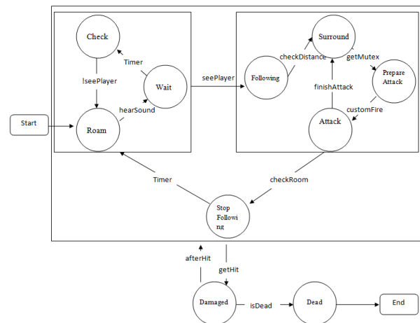
Gambar 1. Diagram FSM dari enemy
