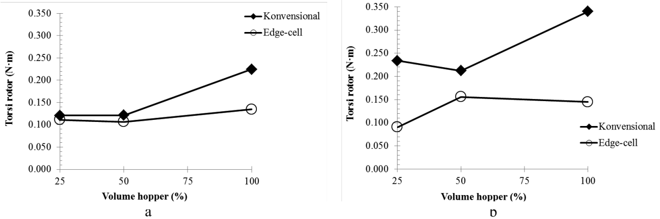
Gambar 7. Perbandingan kebutuhan torsi kedua tipe penjatar pupuk pada pupuk urea bukaan selubung 100%; (a) 15 RPM dan (b) 35 RPM
