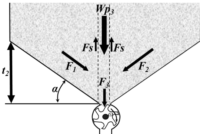
Gambar 14. Koreksi perhitungan pendugaan gaya berat pupuk dalam hopper
