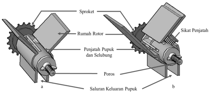
Gambar 5. Penjajah pupuk; (a) konvensional dan (b) edge-cell
