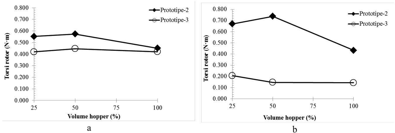
Gambar 10. Perbandingan kebutuhan torsi kedua tipe penjajah pupuk pada pupuk TSP; (a) 15 RPM dan (b) 35 RPM
