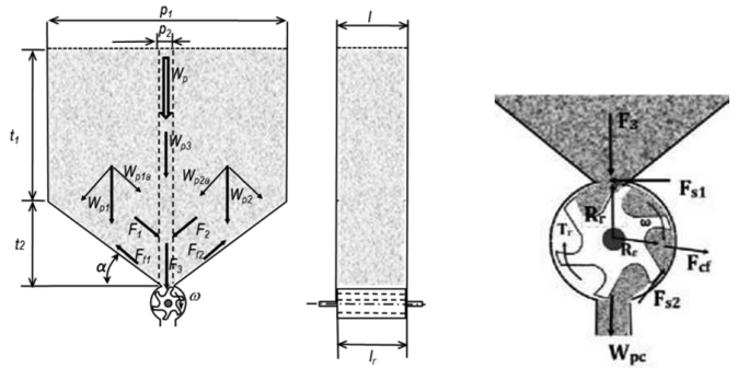
Gambar 2. Analisis pendugaan torsi rotor konvensional
