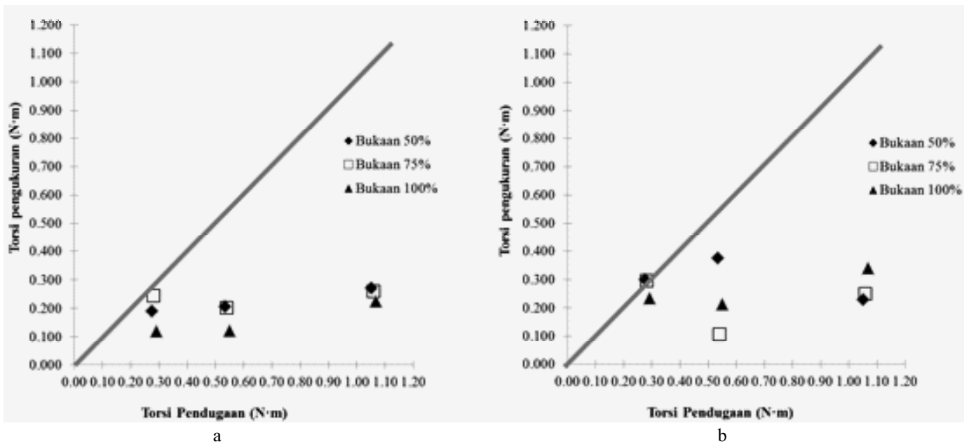
Gambar 13. Hasil validasi model penjataan pupuk urea tipe edge-cell ; (a) 15 RPM, (b) 35 RPM
