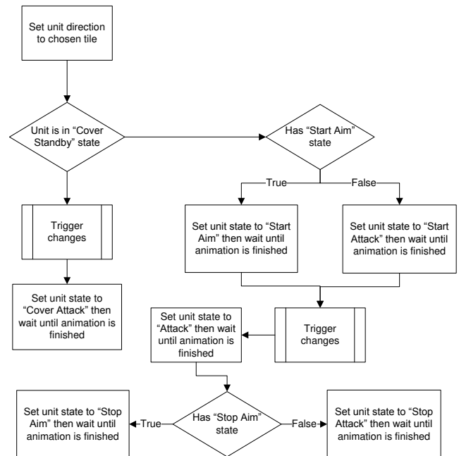
Gambar 5. Skema dari animasi Attack
