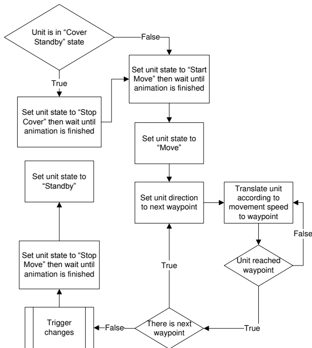
Gambar 4. Skema dari animasi Move
