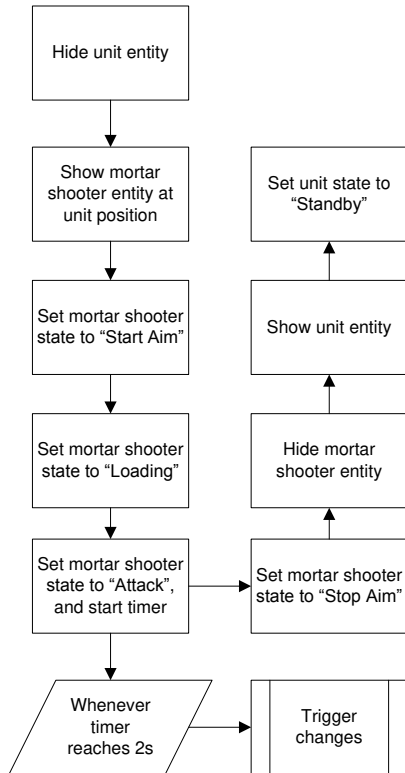
Gambar 6. Skema dari animasi Attack
