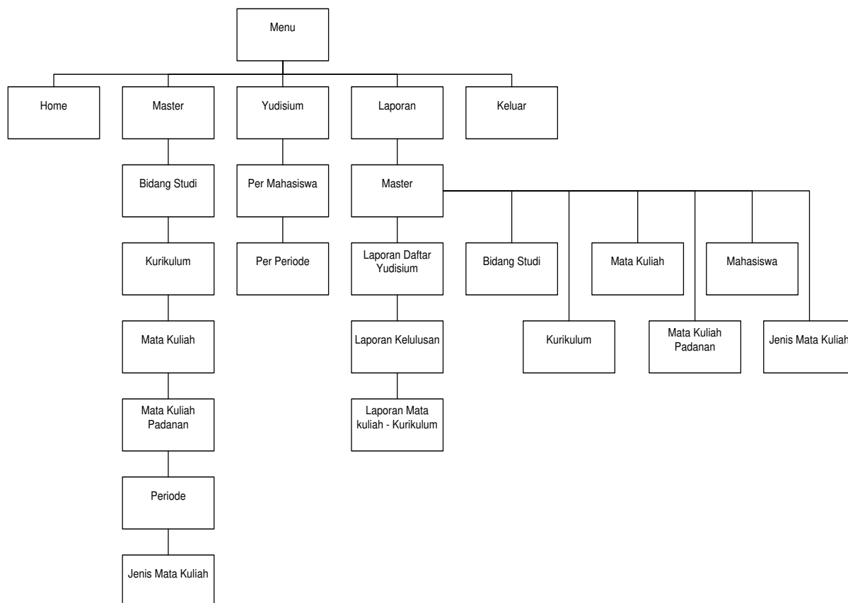
Gambar 4. Desain Menu
