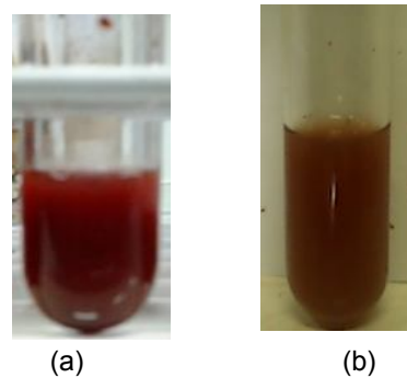
Gambar 6. Larutan dari serbuk pigmen dengan (a) maltodekstrin 5% dan (b) maltodekstrin 10%.
