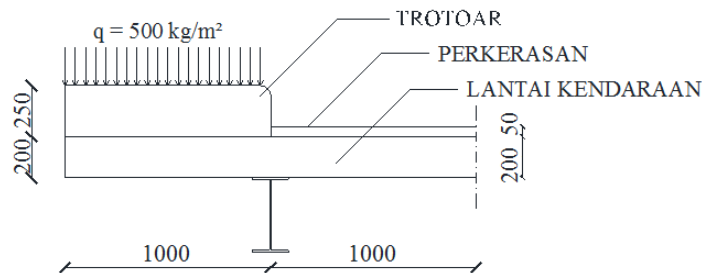
Gambar 3. Pembebanan Pada Gelagar Tepi
