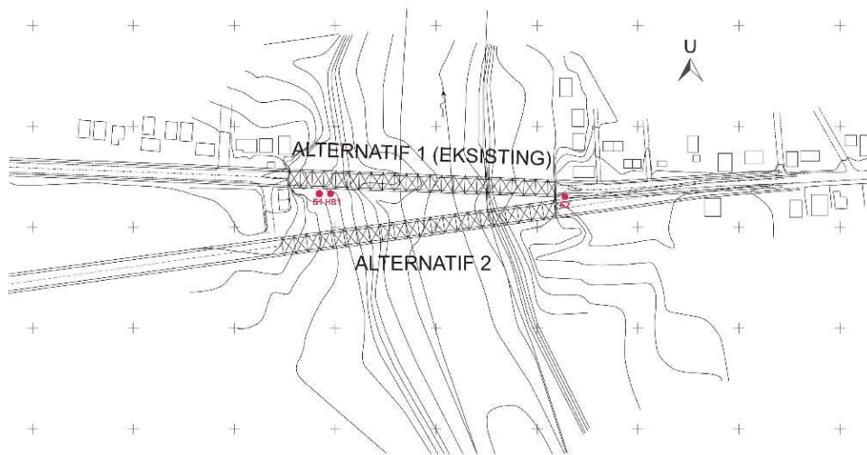
Gambar 1. Denah Jembatan Alternatif 1 dan 2
