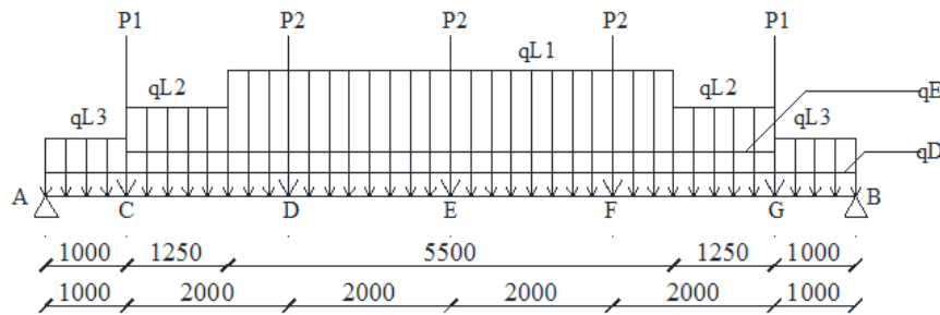
Gambar 6. Pembebanan Pada Perhitungan Shear Connector
