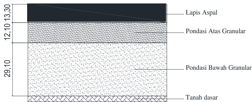
Gambar 10. Struktur Lapisan Tebal Perkerasan
