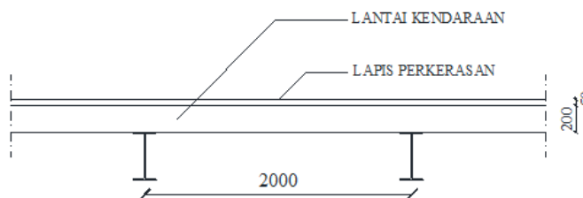
Gambar 4. Penampang Melintang Gelagar Tengah
