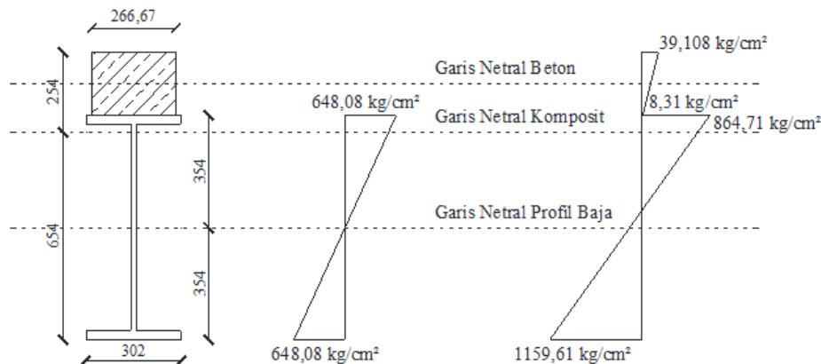
Gambar 5. Diagram Tegangan Sebelum Dan Sesudah Komposit
