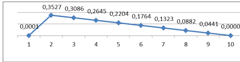
Gambar 9. Output SAP 2000 garis pengaruh
