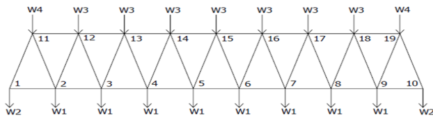
Gambar 8. Pola Pembebanan Beban Mati
