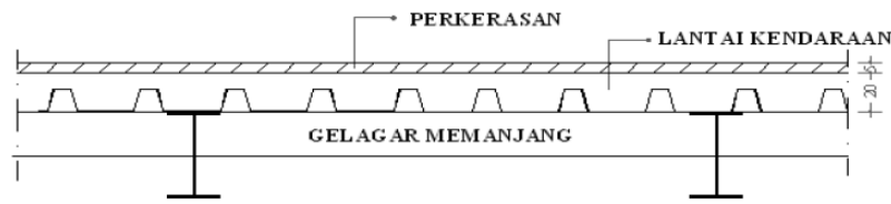
Gambar 2. Perencanaan Pelat Lantai Jembatan
