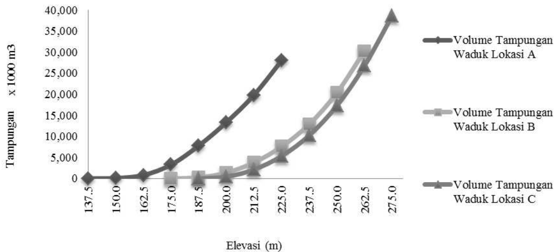
Gambar 5. Grafik Perbandingan Kapasitas Volume Tampungan Masing-masing Alternatif Lokasi
