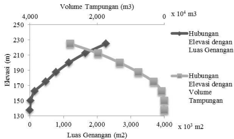
Gambar 2. Kurva Tampungan di Lokasi A
