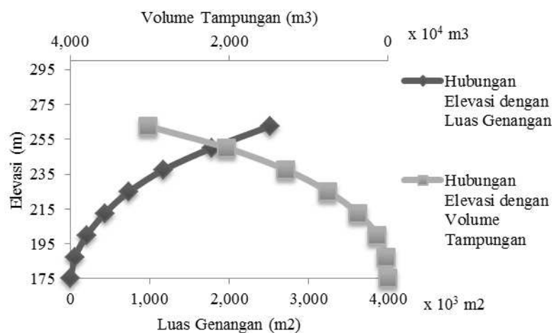
Gambar 3. Kurva Tampungan di Lokasi B
