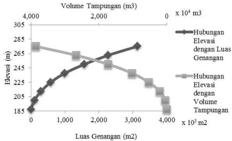
Gambar 4. Kurva Tampung di Lokasi C
