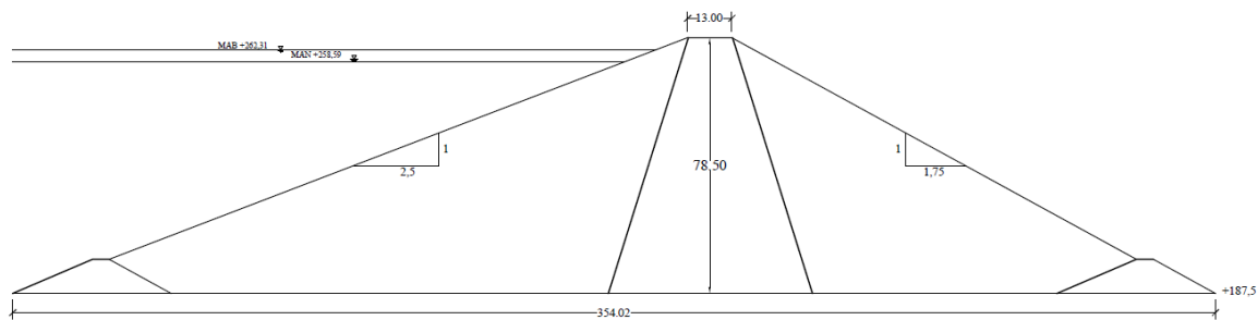
Gambar 9. Sketsa Penentuan Tinggi, Lebar dan Panjang Dasar
