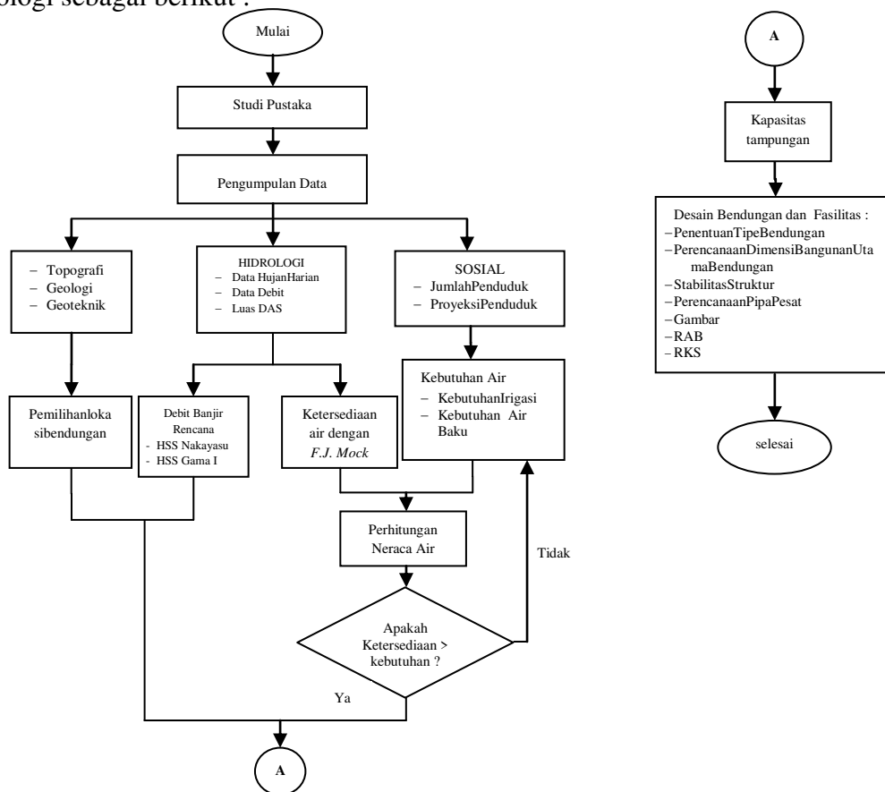
Gambar 1. Bagan Alir Metode Perencanaan.
