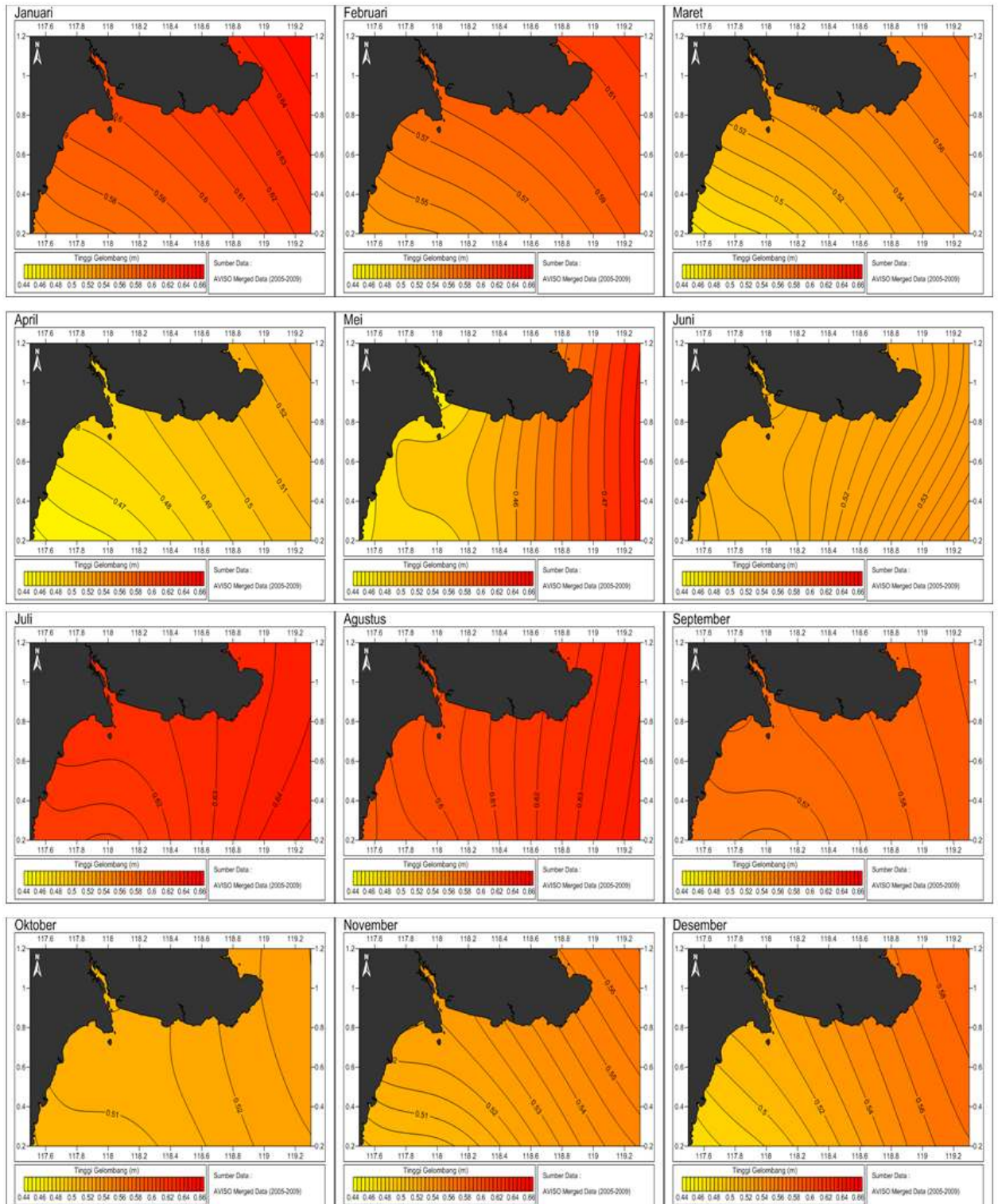
Gambar 2. Pola gelombang bulanan (Januari – Desember) di perairan sepanjang pesisir Kabupaten Kutai Timur
