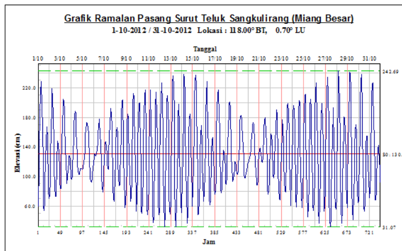
Gambar 6. Pola pasang surut selama satu bulan (Oktober 2012) di perairan sekitar pesisir Kabupaten Kutai Timur
