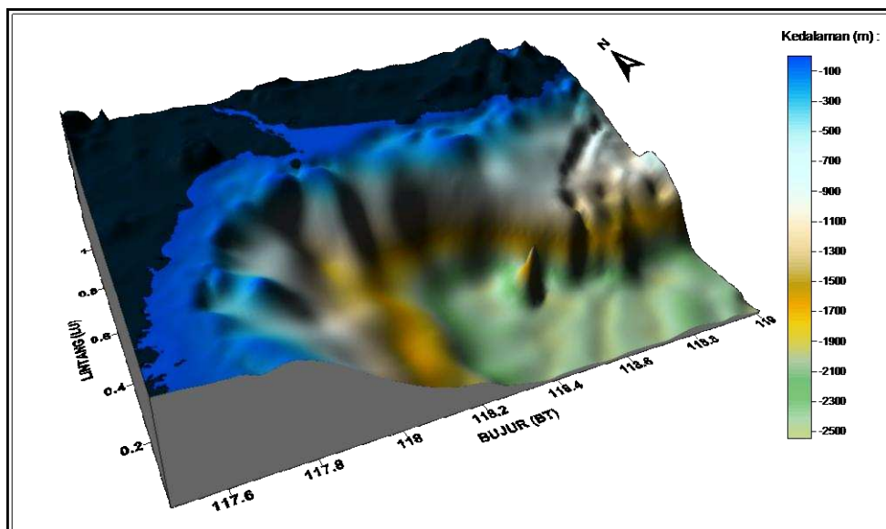
Gambar 3. Profil kedalaman perairan secara 3D sepanjang pesisir Kabupaten Kutai Timur
