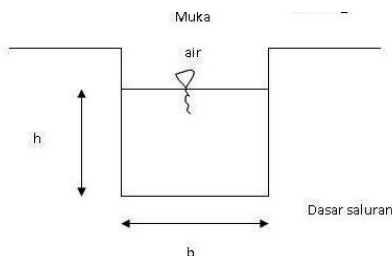
Gambar 4. Penampang saluran rencana (persegi)
