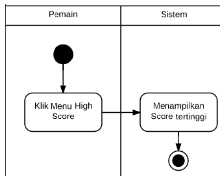
Gambar 5. Activity Diagram Pemilihan Menu High Score
