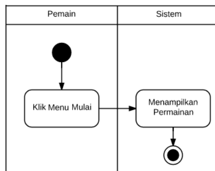
Gambar 4. Activity Diagram Pemilihan Menu Mulai
