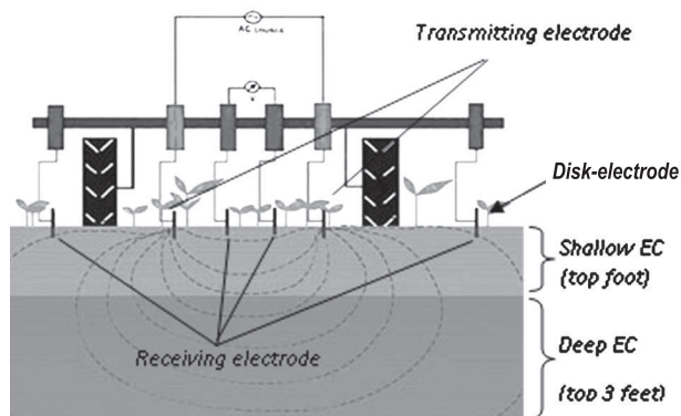
Gambar 2. Cara kerja pengukuran EC tanah pada instrumen Veris 3100.
