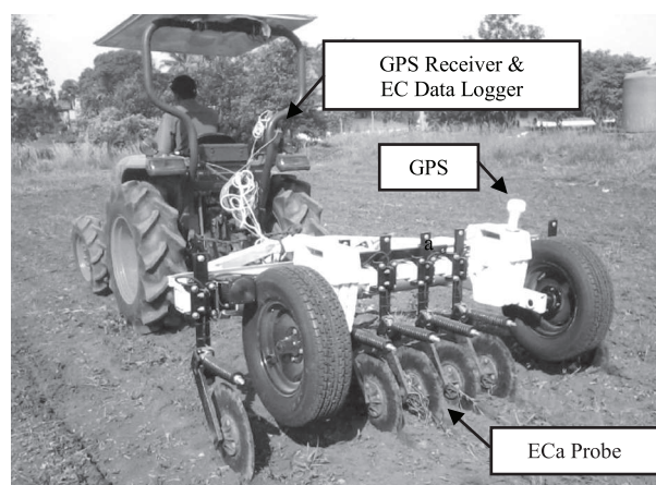
Gambar 4. Instrumen Veris 3100 & GPS ditarik dengan traktor.
