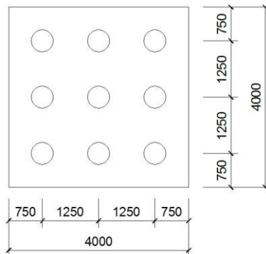
Gambar 10. Pondasi P1
