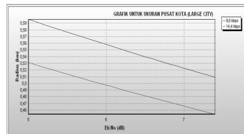
Gambar 4. Grafik Hubungan antara E_b/N_o terhadap radius cakupan pada daerah suburban untuk pusat kota dengan CM=3
