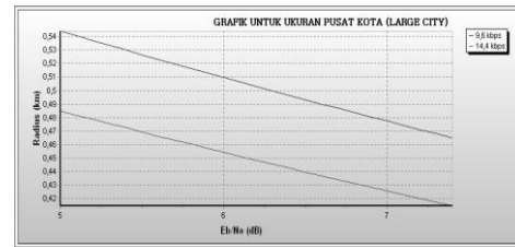
Gambar 3. Grafik Hubungan antara E_b/N_o terhadap radius cakupan untuk daerah berjenis urban di pusat kota dengan nilai CM=3
