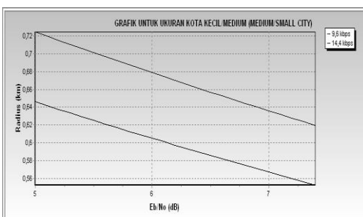
Gambar 6. Grafik Hubungan antara E_b/N_o terhadap radius cakupan pada daerah suburban untuk kota kecil-sedang dengan CM=0
