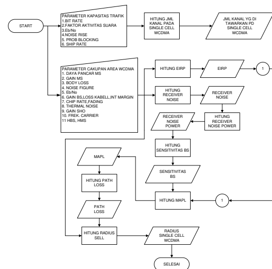
Gambar 1. Diagram alir simulasi menggunakan Delphi untuk melihat dan menganalisis pengaruh E_b/N_o terhadap Jumlah Kanal dan Cakupan WCDMA
