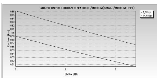
Gambar 6. Grafik Hubungan antara E_b/N_o terhadap radius cakupan pada daerah urban untuk kota kecil-sedang dengan CM=0
