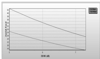
Gambar 2. Grafik hubungan antara nilai E_b/N_o dengan jumlah kanal yang ditawarkan
