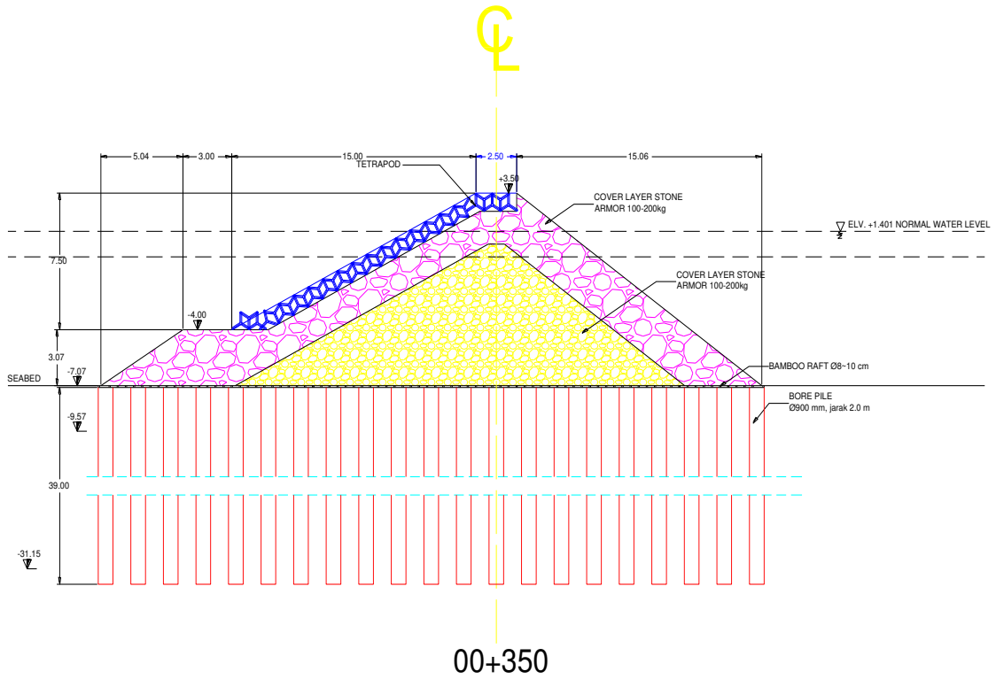
Gambar 12. Permodelan Solusi Perkuatan Tanah 3
