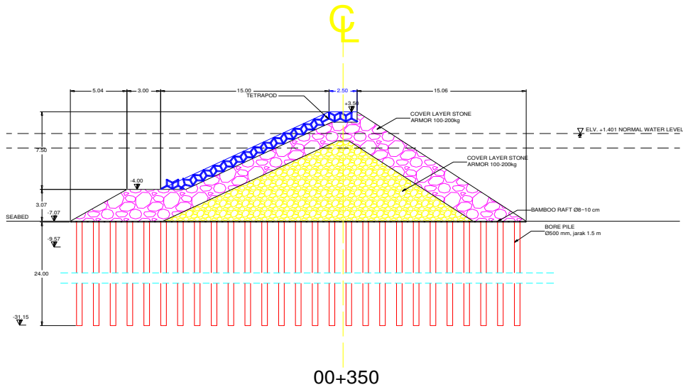
Gambar 11. Permodelan Solusi Perkuatan Tanah 2
