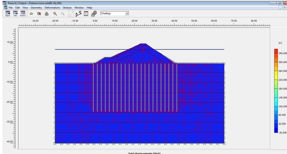
Gambar 17. Output Shading Solusi Perkuatan Tanah 4
