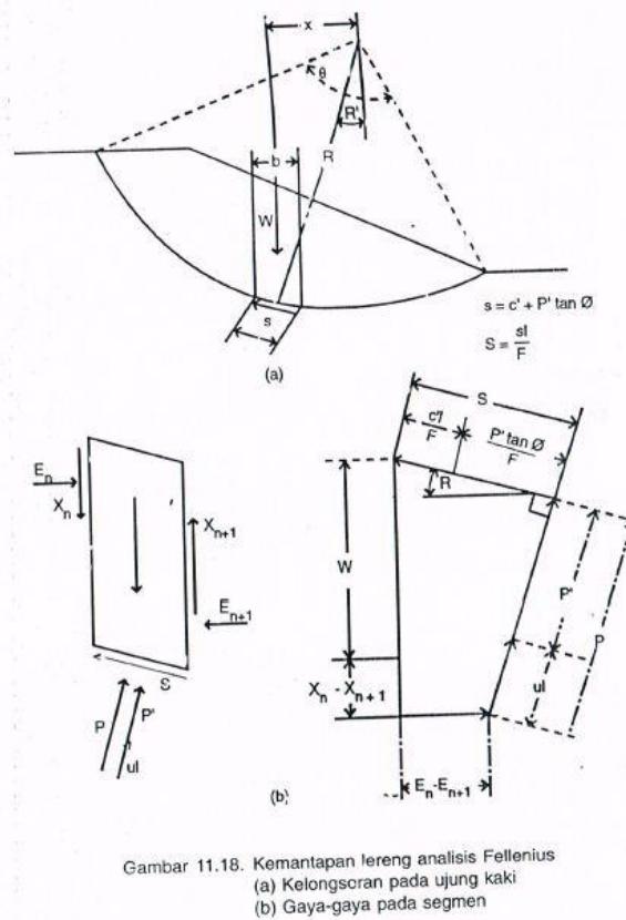
Gambar 3. Sistem gaya pada cara Fellenius
