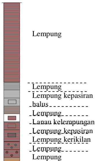
Gambar 6. Stratifigrasi Tanah
