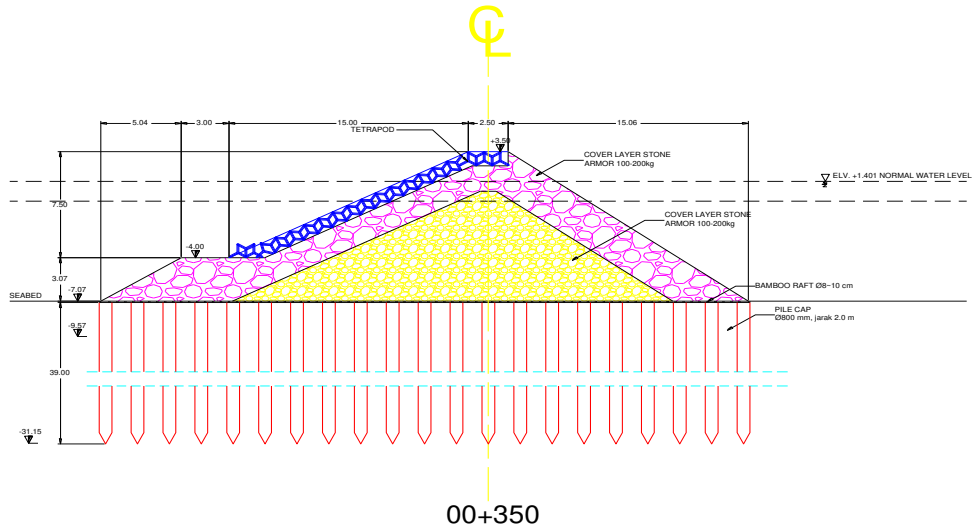
Gambar 10. Permodelan Solusi Perkuatan Tanah 1
