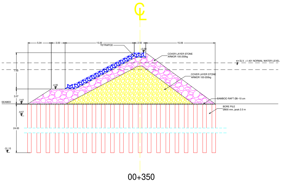
Gambar 13. Permodelan Solusi Perkuatan Tanah 4
