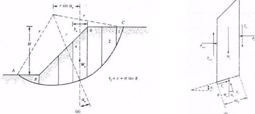
Gambar 2. Gaya – gaya yang bekerja pada irisan bidang longsor
