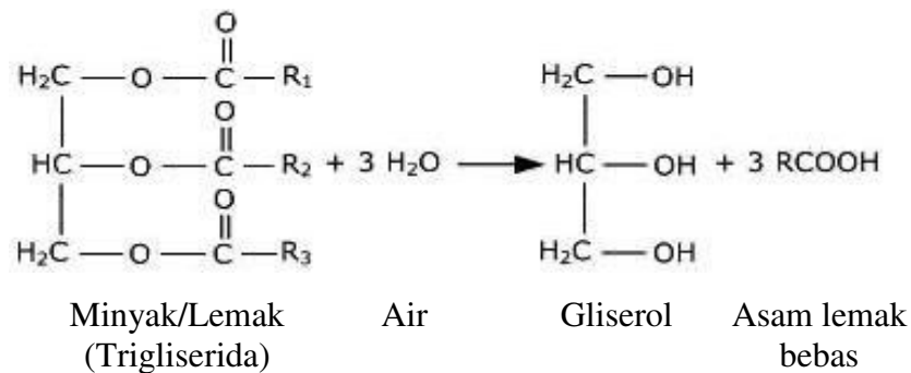
Gambar 2. Hidrolisis Trigliserida
