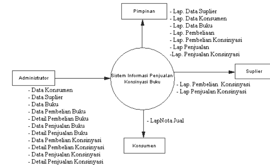
Gambar 1. Diagram Konteks SI Penjualan Buku
