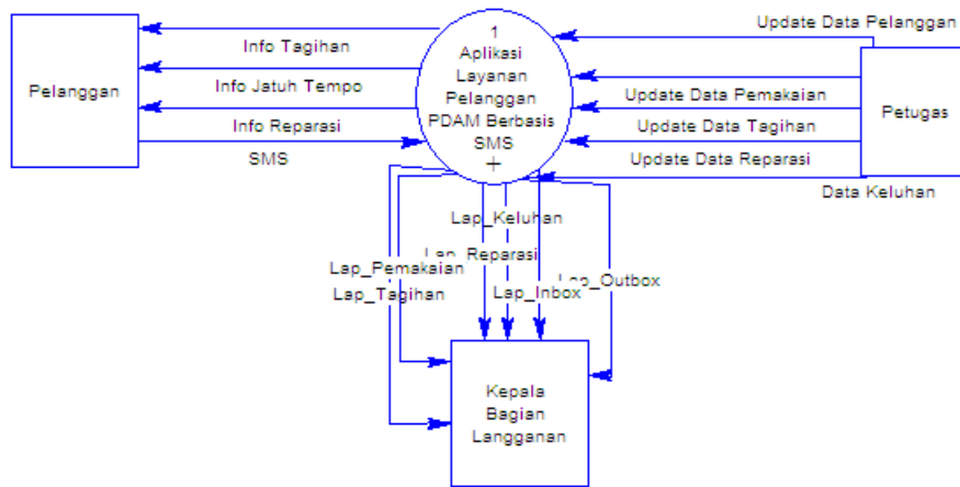
Gambar 1. Diagram Konteks
