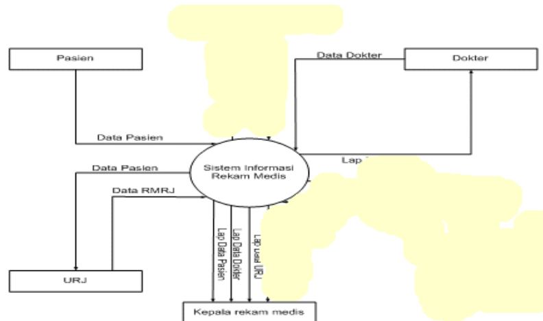
Gambar 1. Diagram konteks
