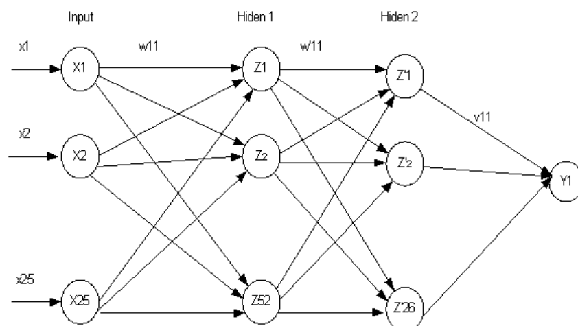
Gambar 2. Arsitektur Jaringan
