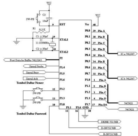
Gambar 4. Rangkaian mikrokontroler unit pendaftaran nomor
